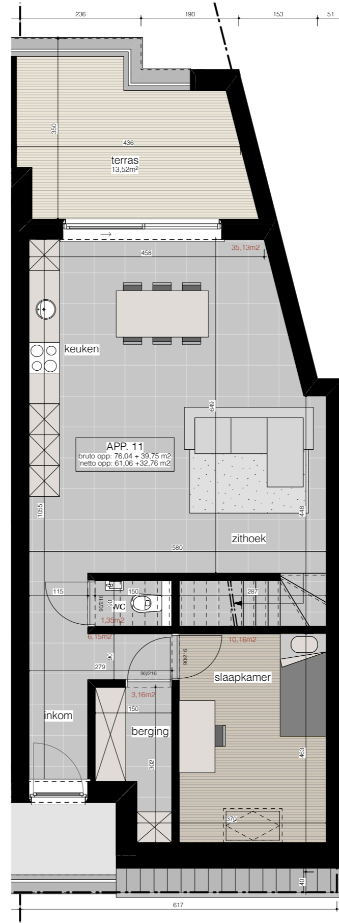
VERDIEPING 2 SCHAAL 1/75
